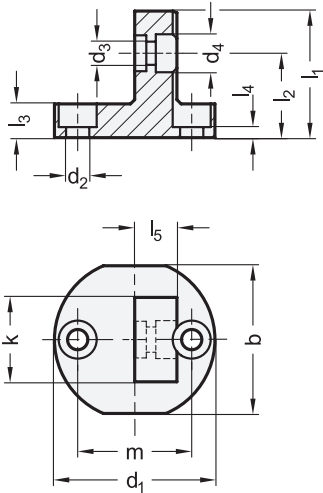
Upínací sada GN 511.1, Typ K
